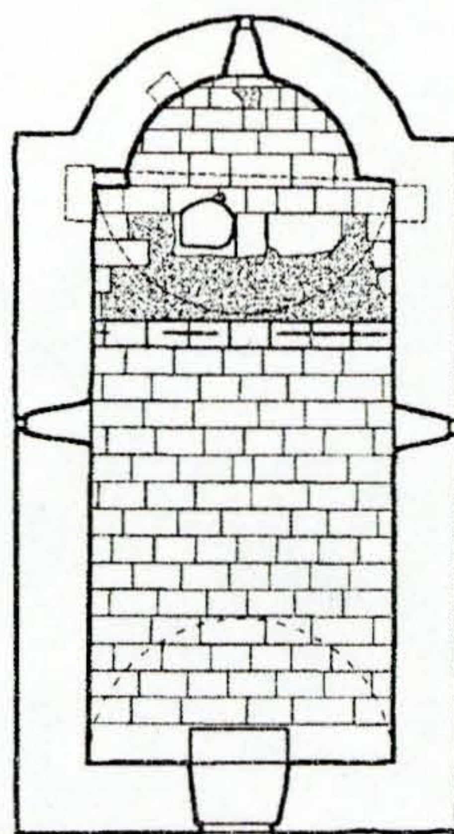
Основа цркве
