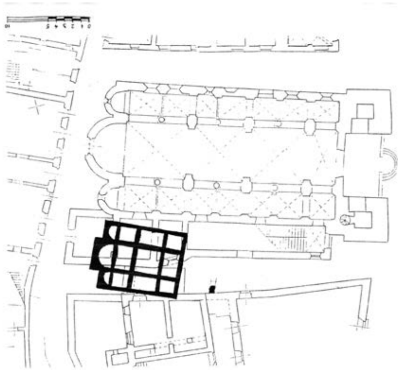
Sl.2 - Osnove crkava Sv. Tripuna iz 9. i 12. vijeka
