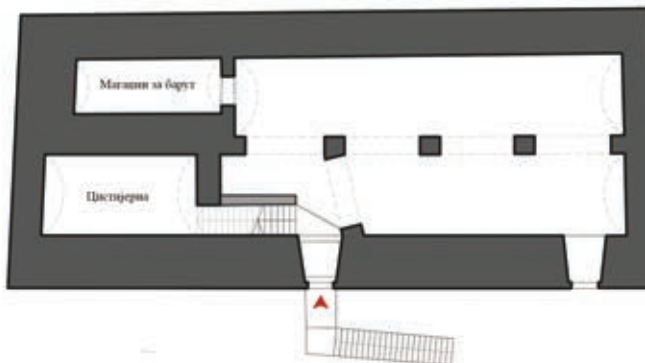
ОСНОВА ПРИЗЕМЉА
