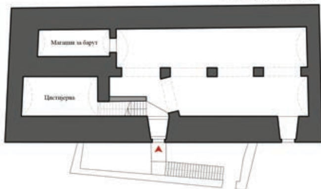
ОСНОВА ПРИЗЕМЉА
