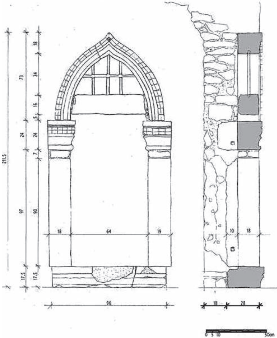
Crtež 5. Gotička monofora (crtež Marina Knežević)
