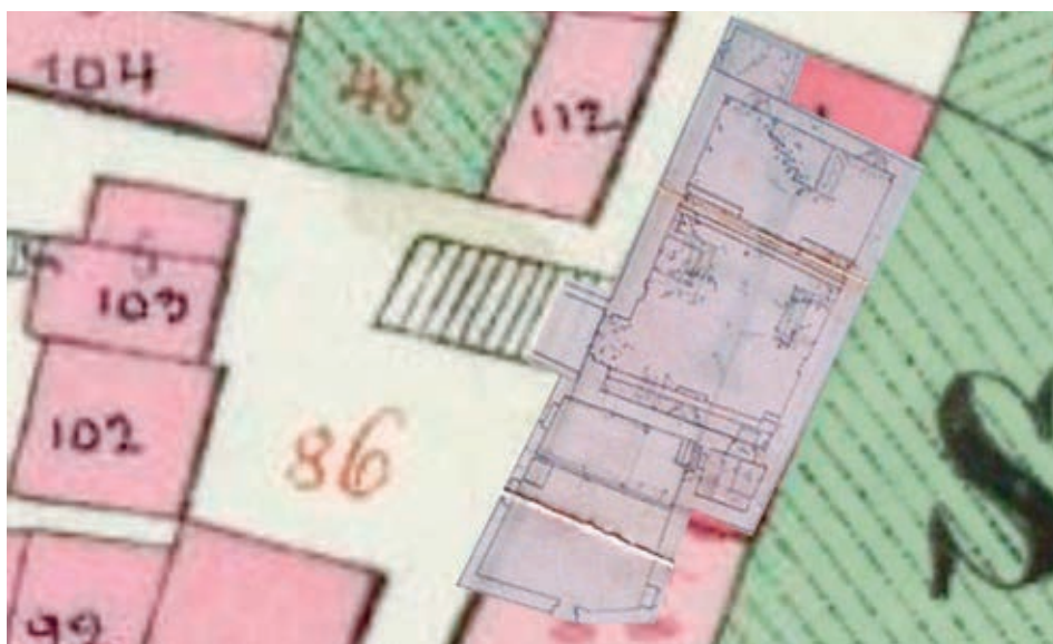
Slika 6. Arhivski crtež, osnova sprata Crkve Sv. Josipa preklapljena sa dijelom katastarsog plana iz 1838. g. na kome su predstavljene analizirane građevine: Crkva Sv. Josipa, zvonik i samostan klarisa
