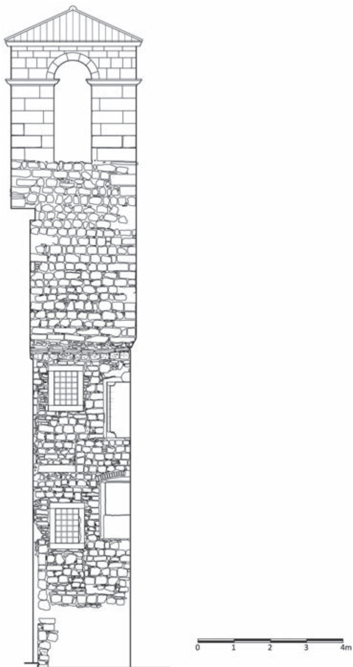
Crtež 3. Zapadni izgled zvonika (crtež Marina Knežević, Katarina Lisavac)
