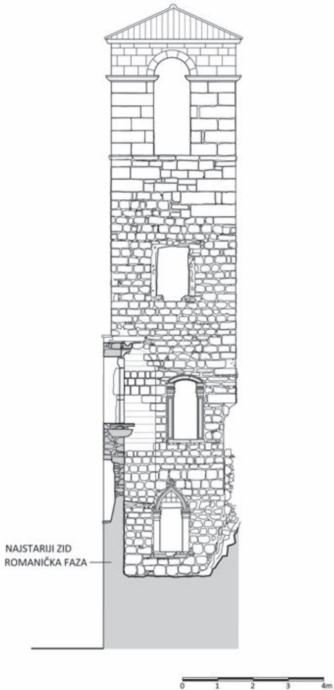
Crtež 4. Južni izgled zvonika (crtež Marina Knežević, Katarina Lisavac)
