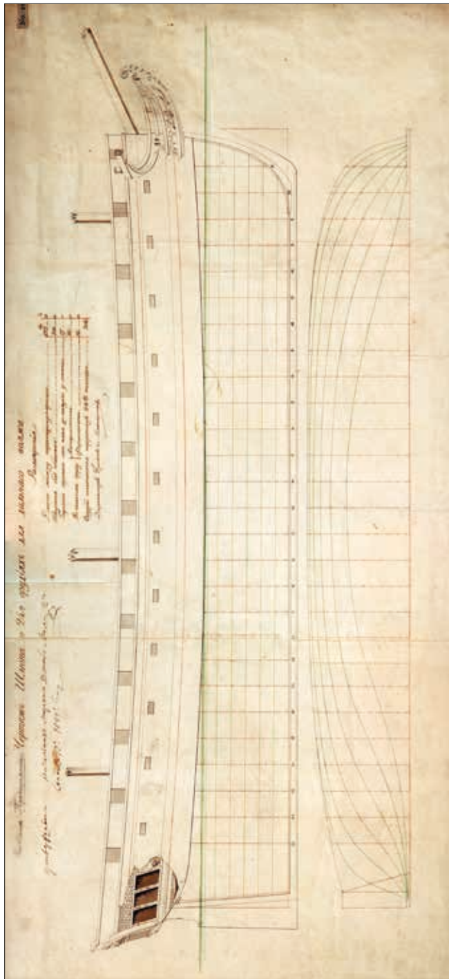
Сл. 2 | Нацрт брода „Предпријатије“, РГАВМФ фонд 327, Опис 1, Ед. Хр. 2918
